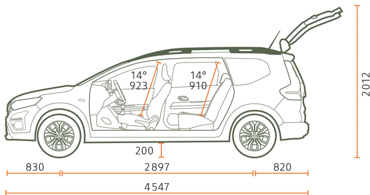
5-MIESTNE - BOČNÝ POHĽAD
