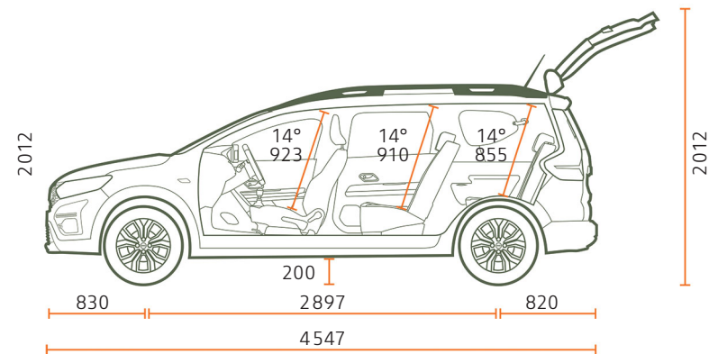
7-MIESTNE - BOČNÝ POHĽAD
