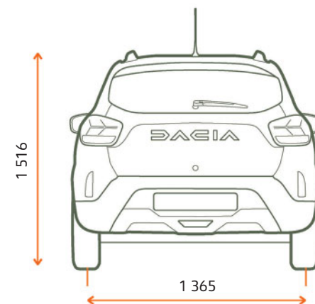
ZADNÝ POHLAD
