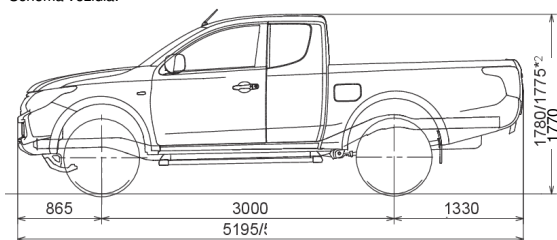
Schéma vozidla:
